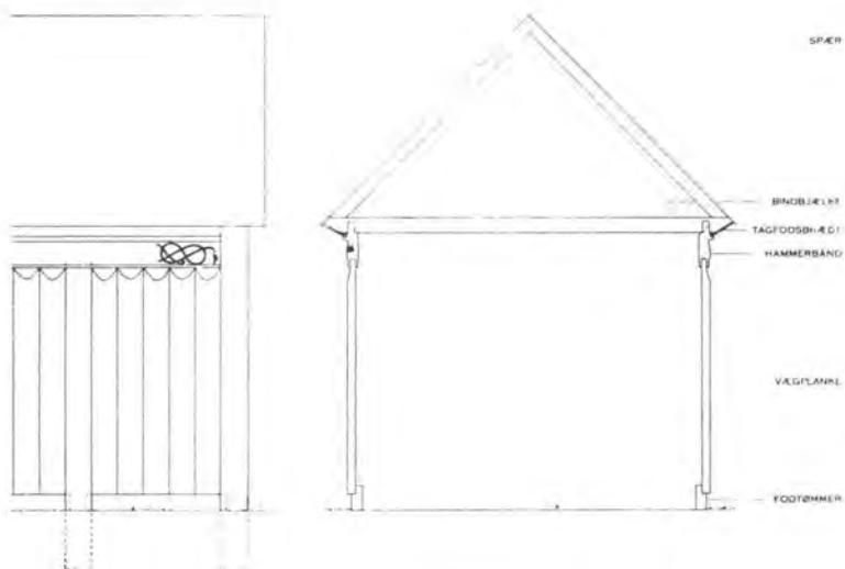
(fig. 9) Opstalt og snit til ansueliggørelse af konstruktionsprincipper m. v. Tegningen må ikke opfattes som et forsøg på rekonstruktion af Høring trækirke.
